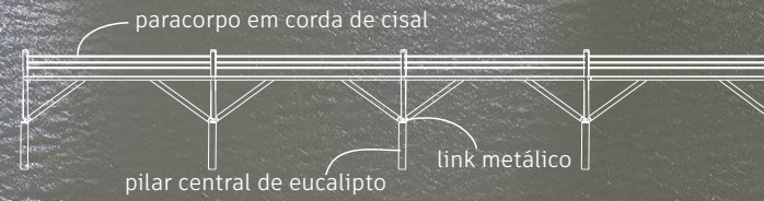
VISTA LATERAL
